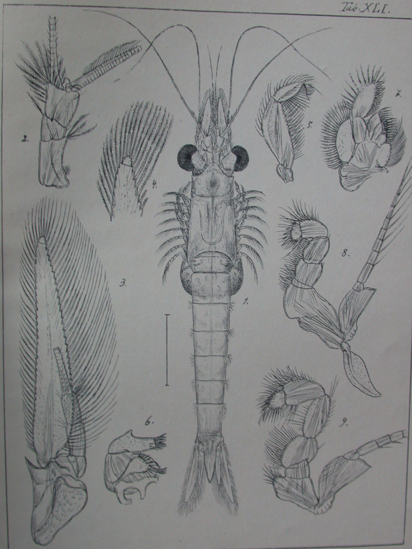
Mysidius grandis (Goës).
