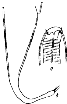
Theristus brachysetosus n. sp. a) Vorderende, b) Schwanz \times 215
