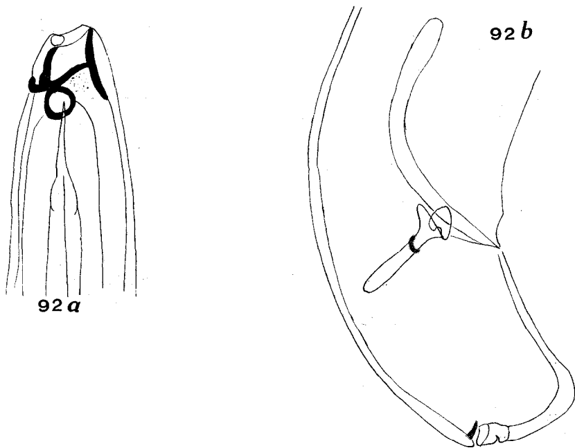
Fig. 92. Siphonolaimus falklandiae n. sp. a. Anterior end, b. Tail and spicules, \times 450
