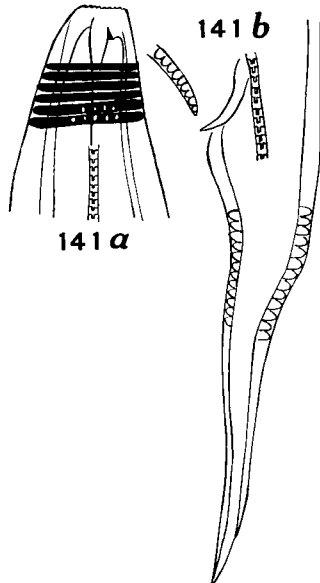
141. Neochromadora notocraspedota ALLGÉN a. Anterior end, \times 450 , b. Tail, \times 270
