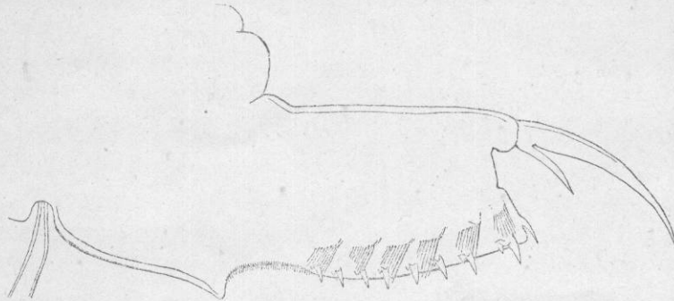
Fig. 11. — Alona Cambouei , ♀, Postabdomen, × 430.
