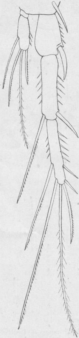
Fig. 8. — Patte de la quatrième paire, \times 430 .
