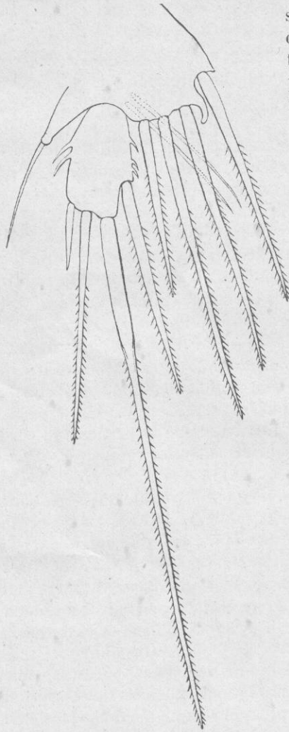
Fig. 9. — Patte de la cinquième paire, longement conique terminé par une soie, lisse comme d'ordinaire. × 60.
