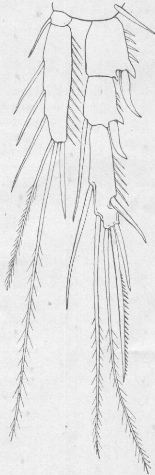
Fig. 7. — Patte de la troisième paire, \times 430 .
