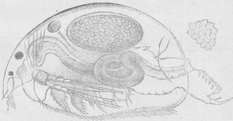
Fig. 10.— Alona Cambouei , ♀, vue de profil, \times 190 ; en haut, à droite, on voit la reticulation à mailles hexagonales et la ponctuation de la carapace, même grossissement.
