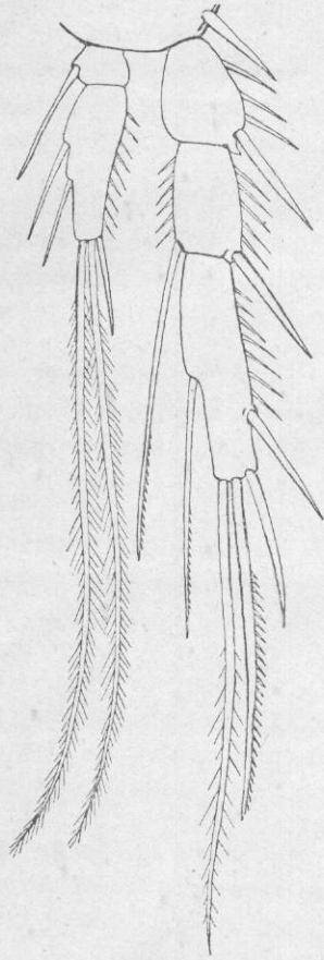
Fig. 6. — Patte de la seconde paire, \times 430 .
