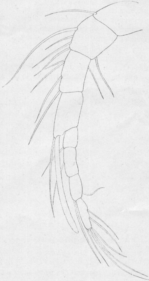
Figure 3. — Antenne de la première paire, \times 430 .
